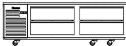
Elevation - TE072HT
